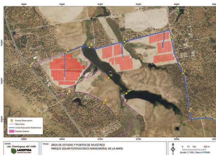
Figura 2. Área del trabajo para el análisis a pequeña escala en relación a las infraestructuras del proyecto y distribución de los puntos de muestreo.
