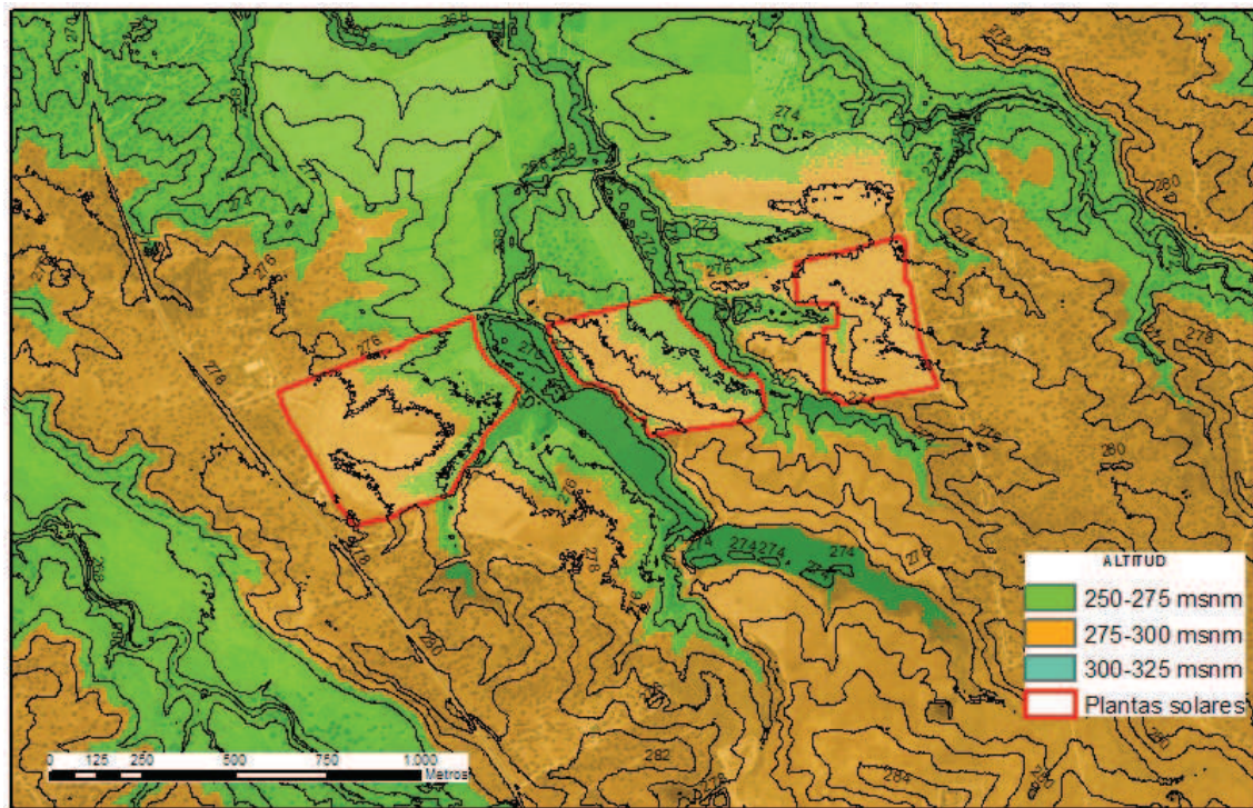
Imagen 3. Detalle de altitudes y curvas de nivel en el entorno de las plantas solares
