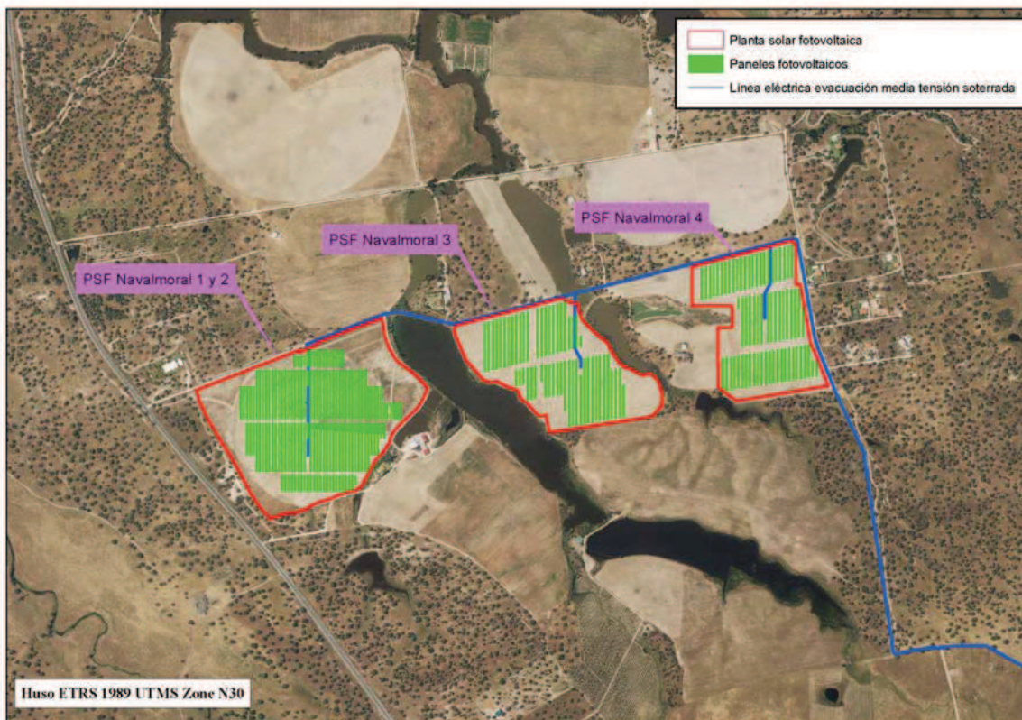
Imagen 3: Localización sobre ortofoto de las PSFV y trazado de zanjas del sistema de evacuación
