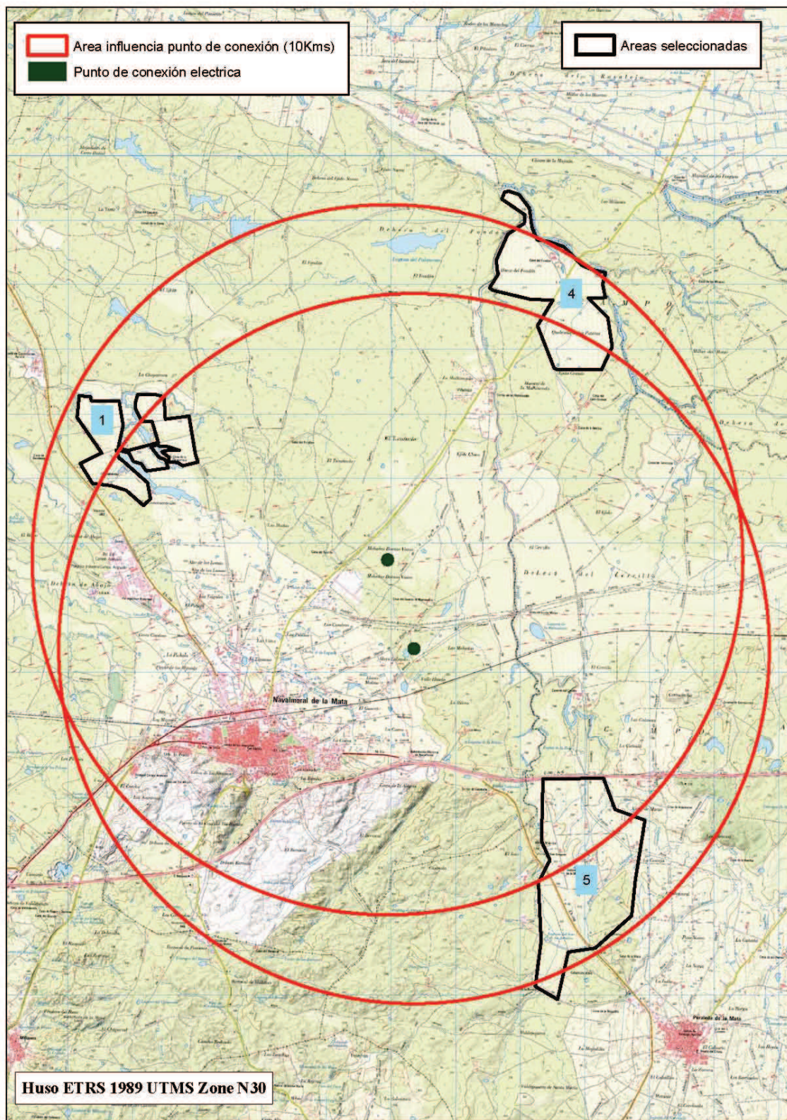
Figura 4: Áreas seleccionadas para instalación de una PSFV en el área de influencia del punto de conexión
