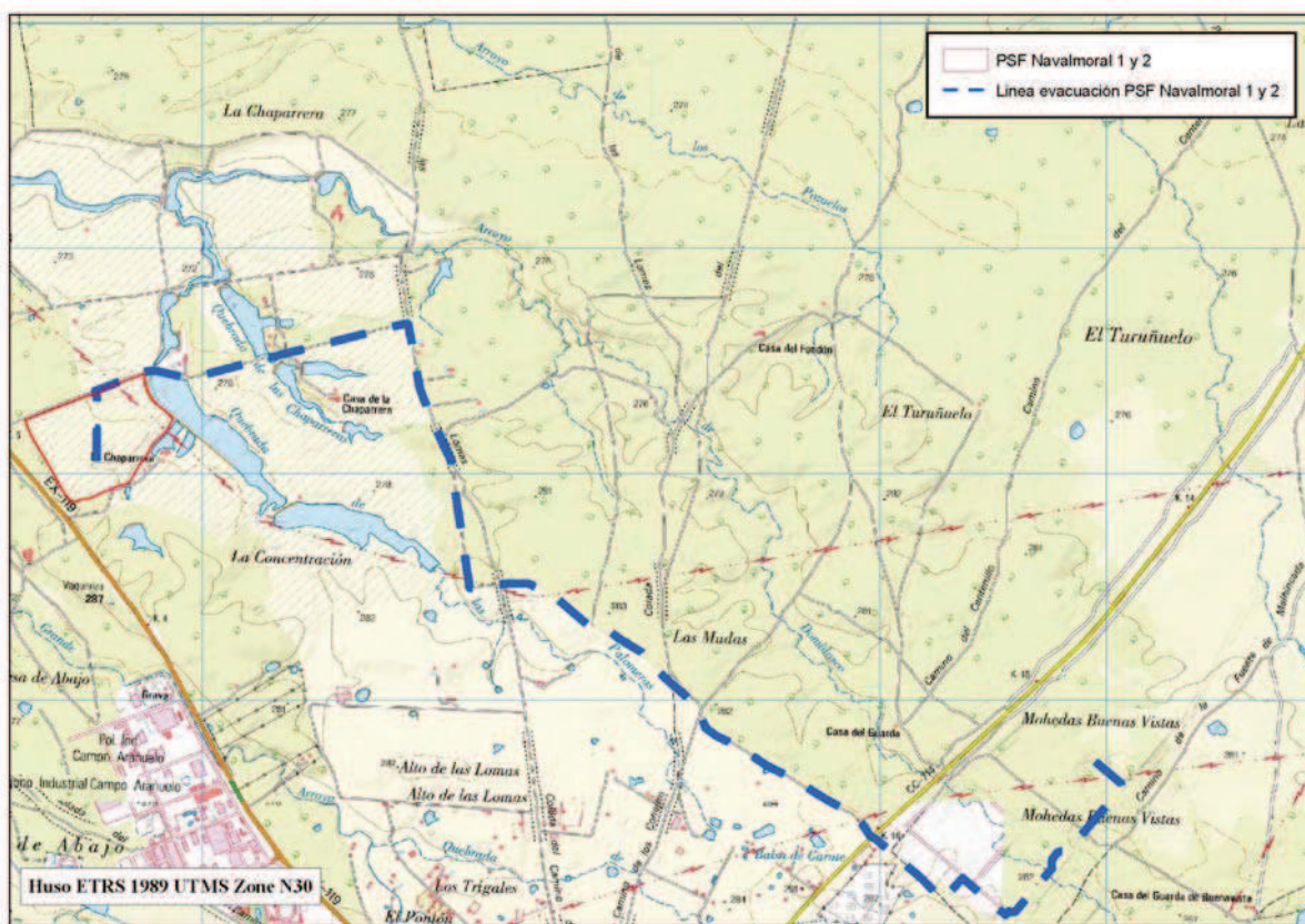
Imagen 4: Trazado LE soterrada de evacuación de la PSFV Navalморal 1 sobre topográfico
