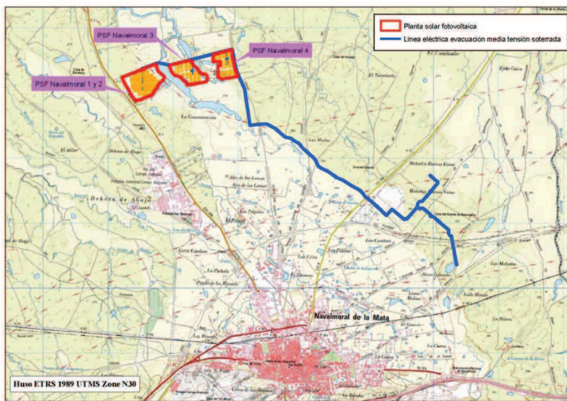
Imagen 2: Localización global del proyecto (entre ellas PSFV Navalmoral 1 y su sistema de evacuación independiente)
