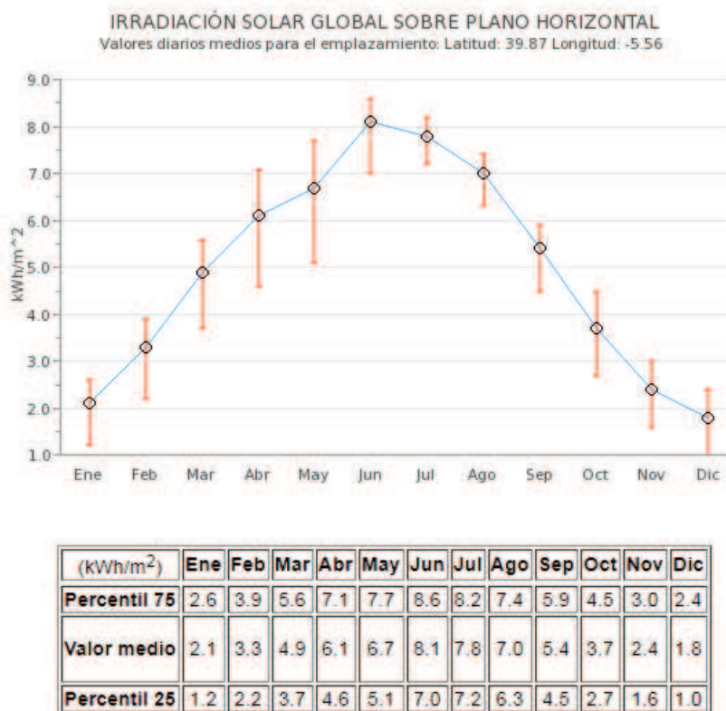
Gráfica 1. Estimación del valor solar mensual
